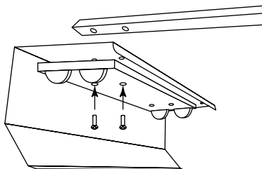
Рисунок 2. Сборка кронштейна
