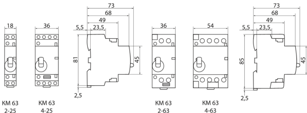
Рисунок 1. Габаритные размеры контакторов, мм
