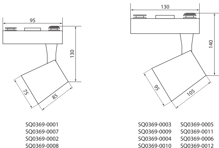
Рисунок 1. Габаритные размеры светильников, мм
