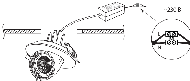
Рисунок 2. Подключение светильника с драйвером к электрической сети
