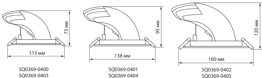
Рисунок 1. Габаритные размеры светильников, мм
