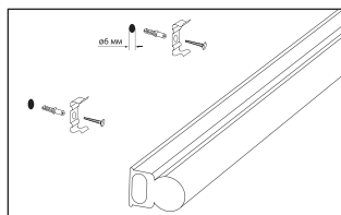
Рисунок 2. Установите клипсы (входят в комплект) для крепления на монтажную поверхность. Защелкните светильник в клипсы.
