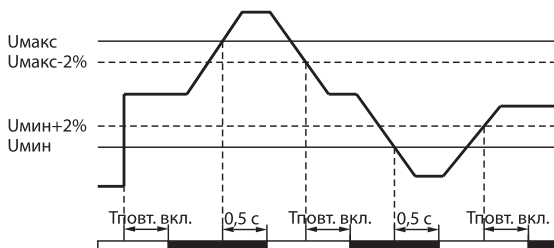
Рисунок 4. Схема работы реле*
