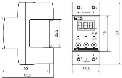
Рисунок 1. Габаритные и установочные размеры, мм
