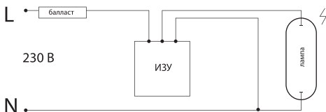
Рисунок 1. Схема подключения
