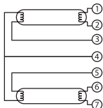
Рисунок 2. Схемы подключения
