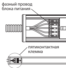
Рисунок 3. Подключение провода питания к клемме
