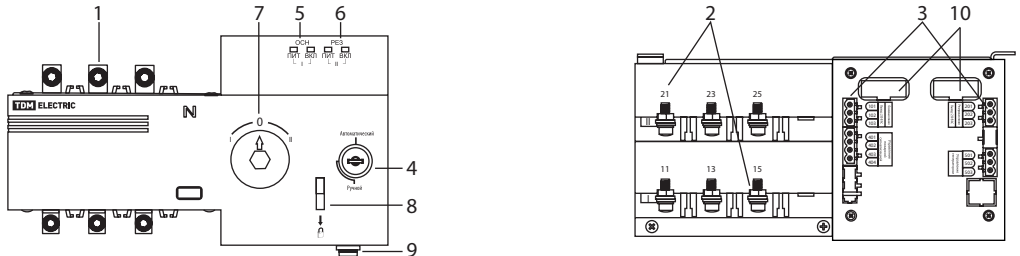
Рисунок 4. Внешний вид АВР-ПН
