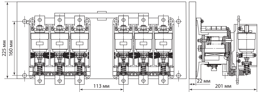
Рисунок 9. Габаритные размеры КВТР-1,14-2,5/250
