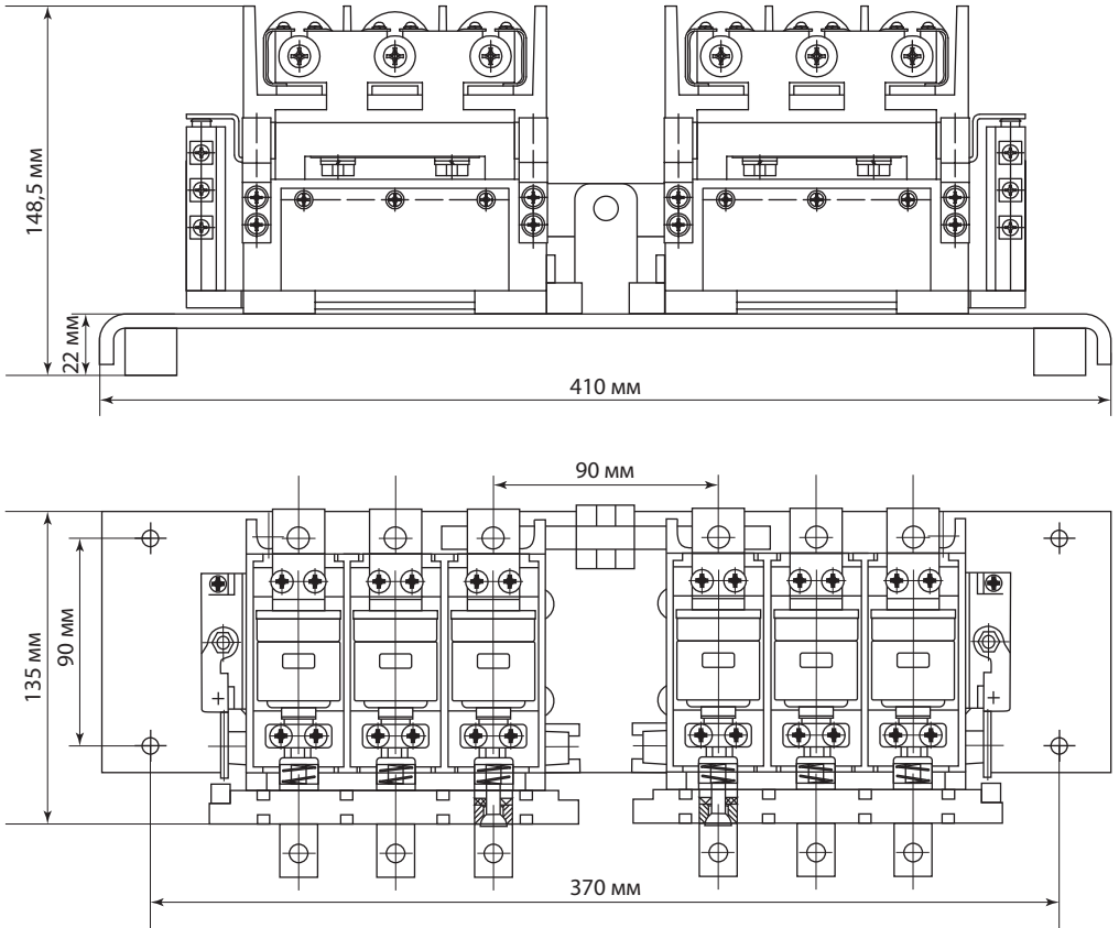
Рисунок 8. Габаритные размеры КВТР-1,14-80/125/160
