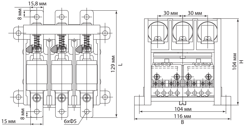
Рисунок 2. Габаритные размеры КВТ-1,14-63
