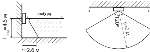
Рисунок 1. Зона обнаружения датчиком движения
