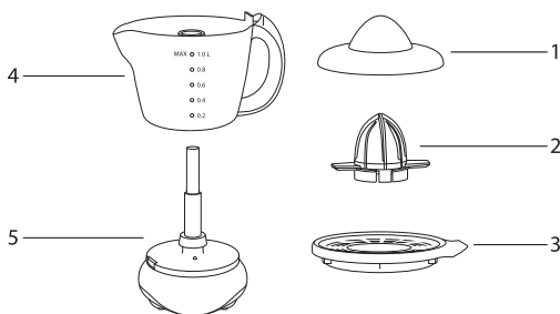
Рисунок 2. Конструкция соковыжималки «Фреш 2»
