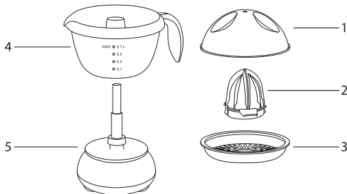
Рисунок 1. Конструкция соковыжималки «Фреш 1»
