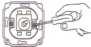
2.5. Установить механизм в отверстие в стене, зафиксировав его стопорными винтами, затянув их до упора.
